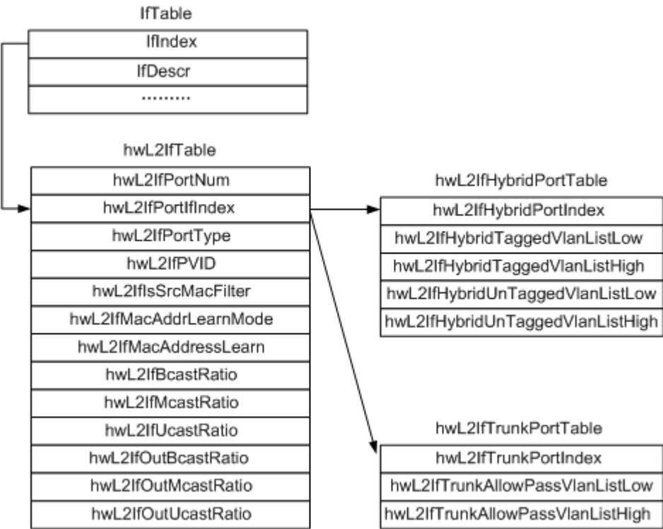
图 69-1 二层端口表、二层 Hybrid 端口表及二层 Trunk 端口表的表间关系图
